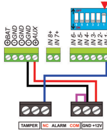
شیاوای دامه‌زاندنی هه‌سته‌هری وایردار به شیاوای یه‌کدانیه‌ی به هاندانی نهرتییی (زونه‌کانی ۱ تا ۶)
