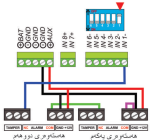
شیاوای دامه‌زاندنی هه‌سته‌هری وایردار به شیاوای زنجیره‌یی به هاندانی نهرتییی (زونه‌کانی ۱ تا ۶)
