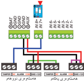
شیاوای دامه‌زاندنی هه‌سته‌هری وایردار به شیاوای زنجیره‌یی به هاندانی نهرتییی (زونه‌کانی ۷ و ۸)
