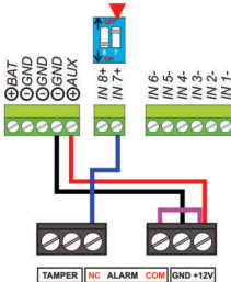
شیاوای دامه‌زاندنی هه‌سته‌هری وایردار به شیاوای یه‌کدانیه‌ی به هاندانی نهرتییی (زونه‌کانی ۷ و ۸)
